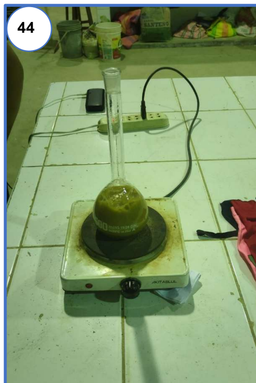
Fotografía N° 43 y N° 44: Muestra del material del agregado fino dentro del frasco volumétrico llenada de agua destilada hasta la marca de enrase y eliminación de burbujas de aire con el uso de cocina eléctrica
