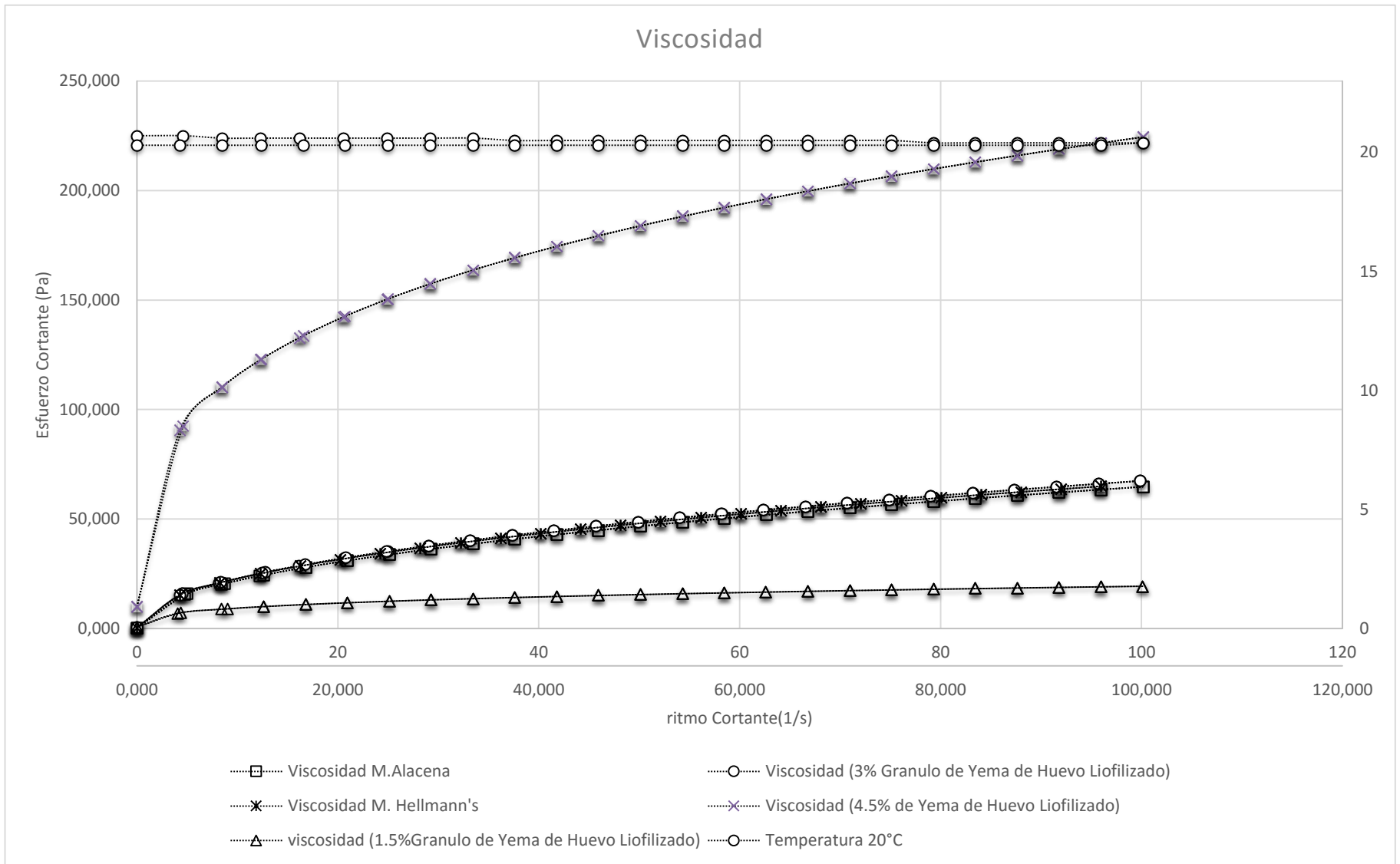
Grafico N° 2: Esfuerzo Cortante (Pa) vs ritmo cortante (1/s).
