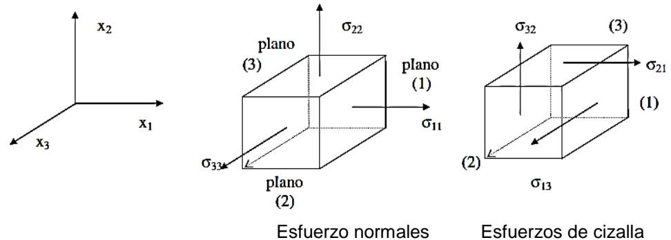
Figura N° 26: componentes del tensor esfuerzo
