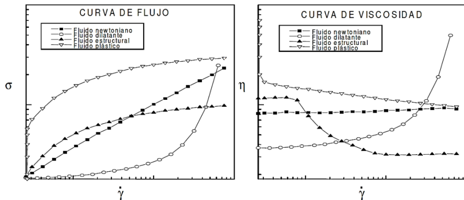
Figura N° 27: Curvas de flujo y viscosidad
