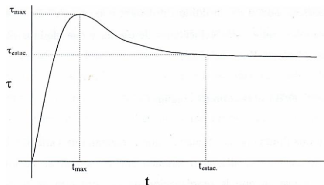
Figura N° 29: Curva característica de un ensayo de flujo transitorio a velocidad de cizalla constante.
