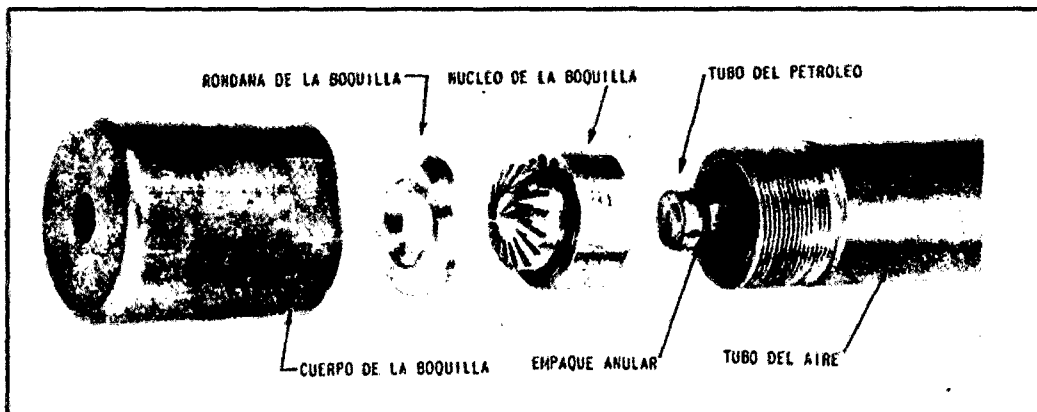
Figura N° 9 Atomizador DISTRAL con inyección de vapor y aire comprimido
