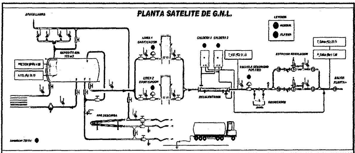
Figura N° 17 Esquema de una Planta Satélite de Regasificación
