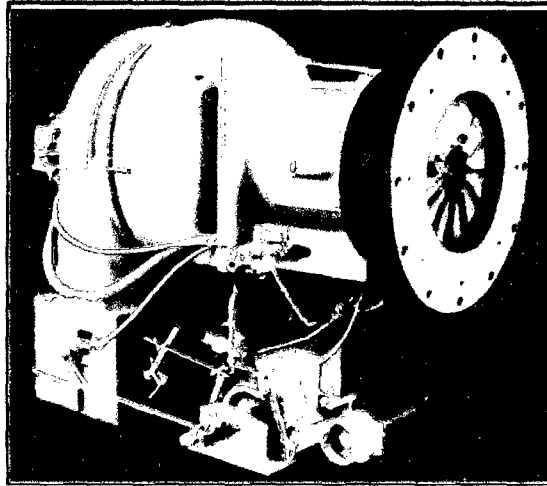
Figura N° 26 Quemador con difusor para Combustible Liquido
