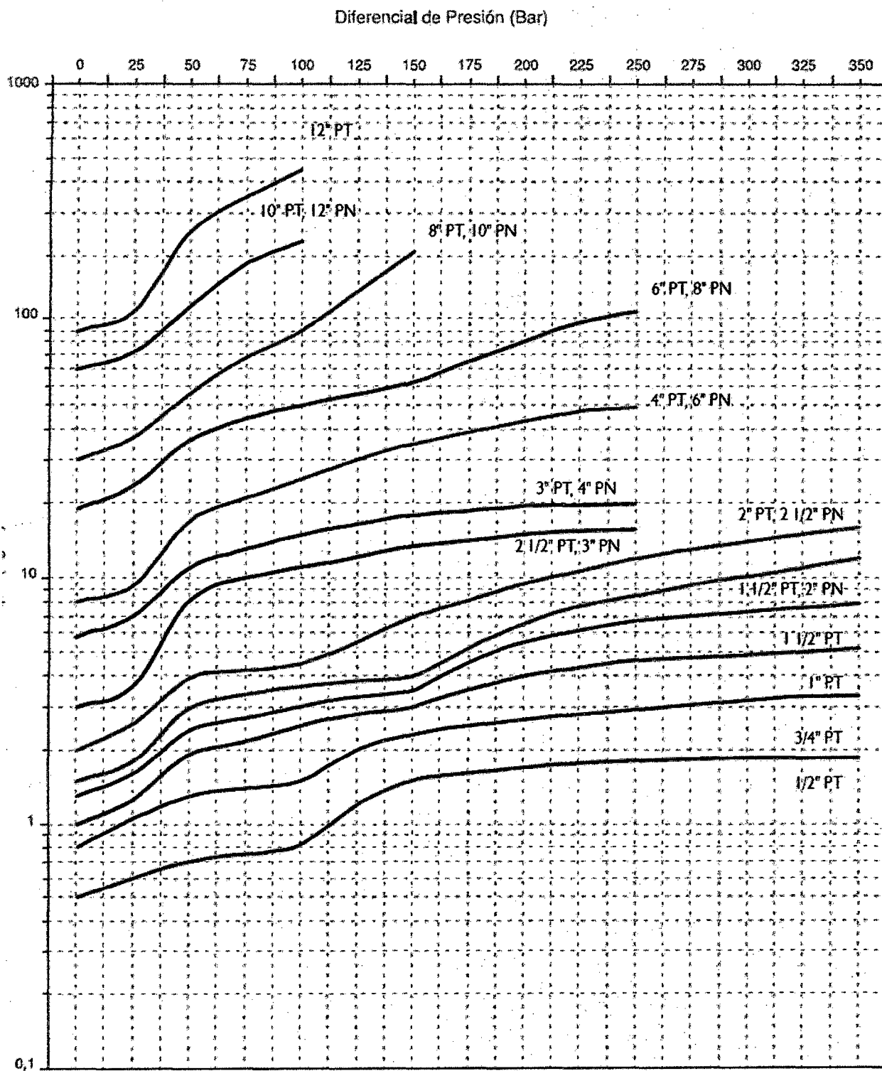
NOMOGRAMA. TORQUE DE ACCIONAMIENTO DE VALVULA ESFEROMATIC
