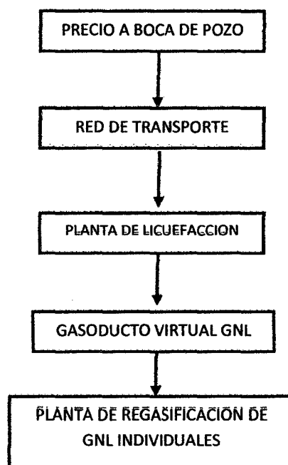
Figura N° 31 Alternativas de suministro de GNL a Chimbote
