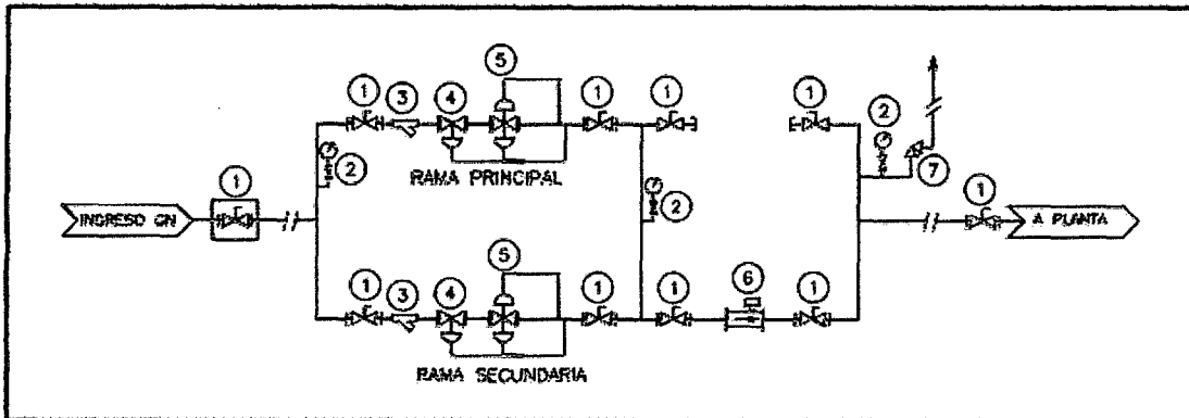
Figura N° 23 ERM de Gas Natural
