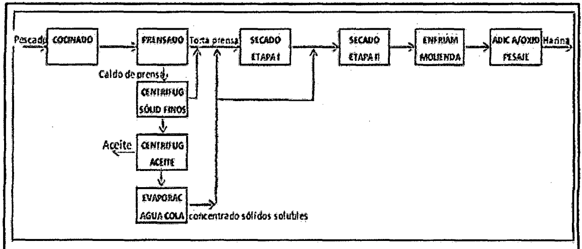
Figura N° 3 Flujograma de Producción de Harina de Pescado
