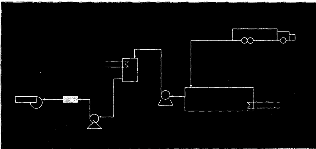
Figura N° 8 Circuito de Petróleo Residual industrial
