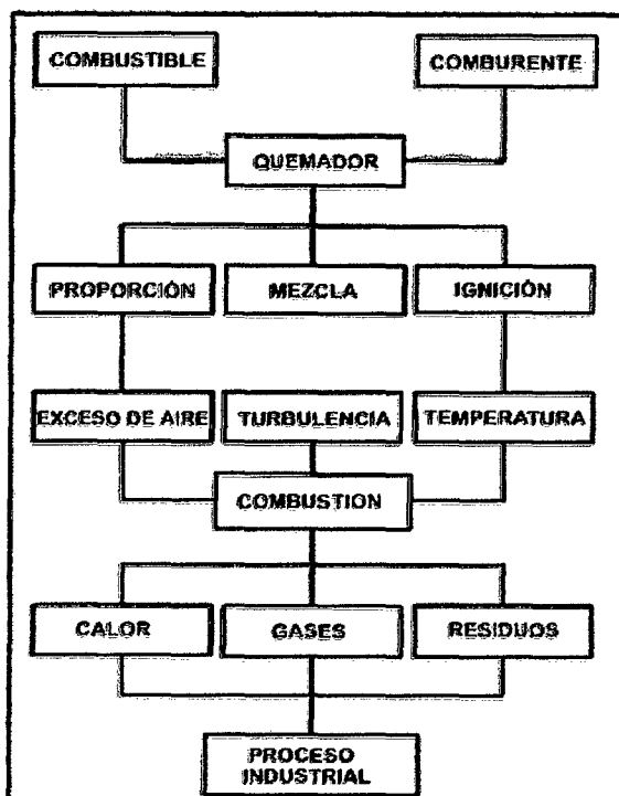
Figura N° 7 Diagrama Esquemático de la combustión industrial
