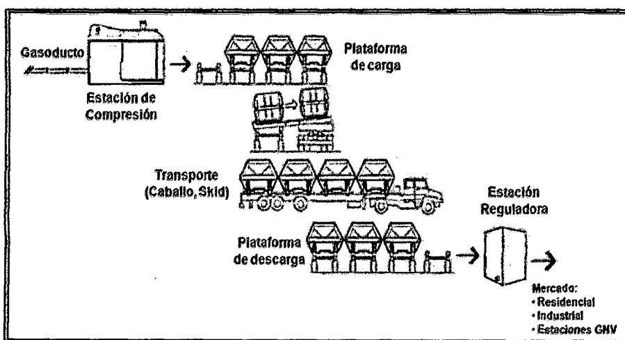
Figura N° 14 Gasoducto Virtual
