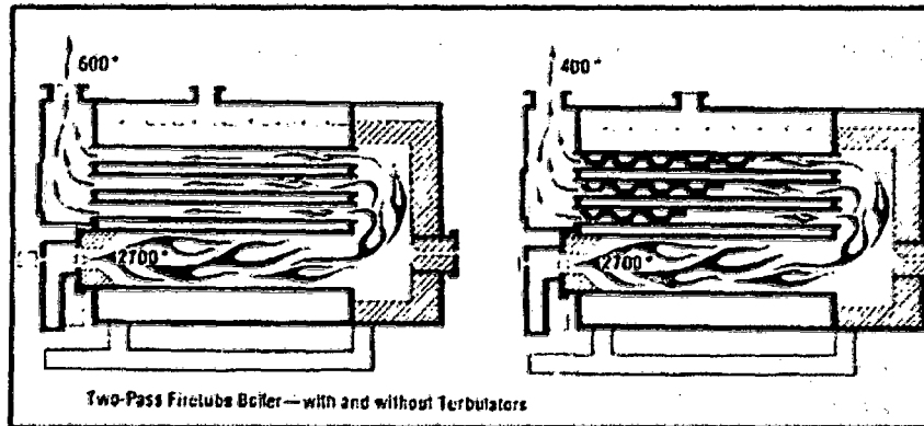
Figura N° 27 Instalación de turbuladores
