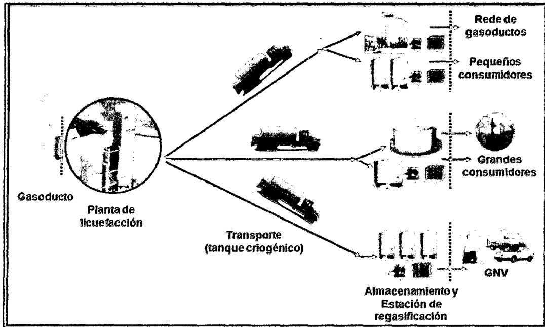
Figura N° 16 Gasoducto Virtual con GNL
