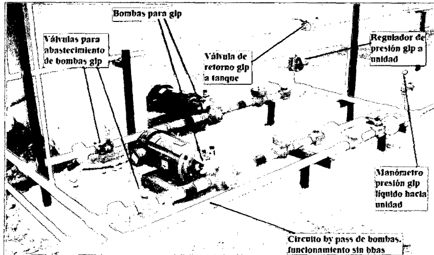
Figura N° 10 Punto de medición de GLP antes de ingresar a planta
